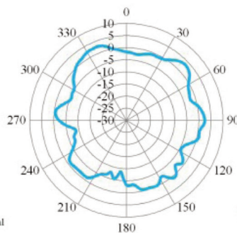
— 3800MHz Vertical
