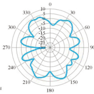
6500MHz Vertical
