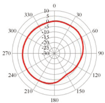
— 3500MHz Horizontal
