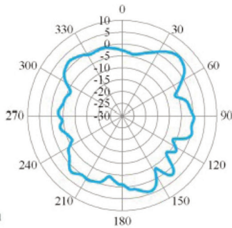
— 3500MHz Vertical
