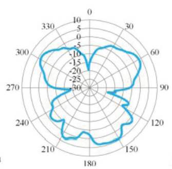
— 2690MHz Vertical
