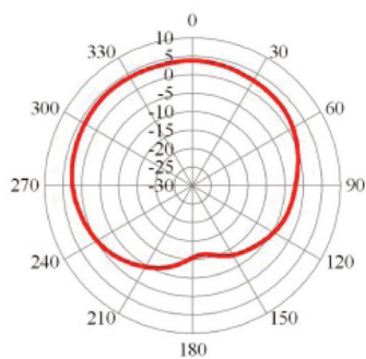
— 3800MHz Horizontal
