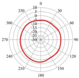
— 2690MHz Horizontal
